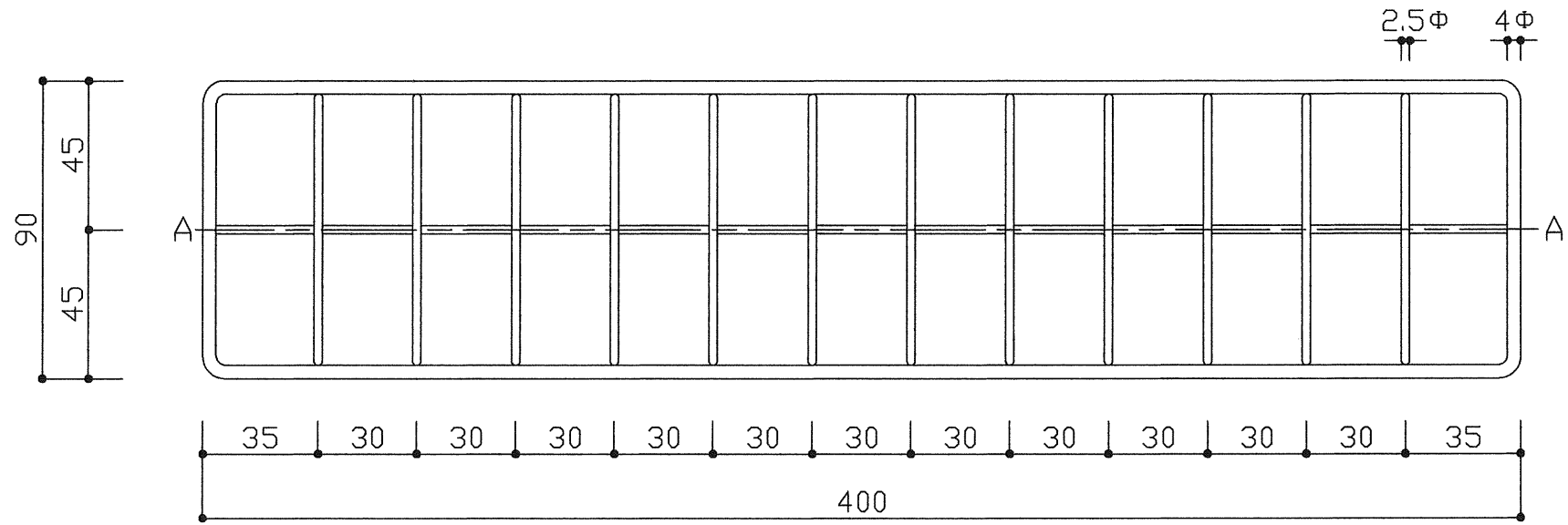
A-A断面図
