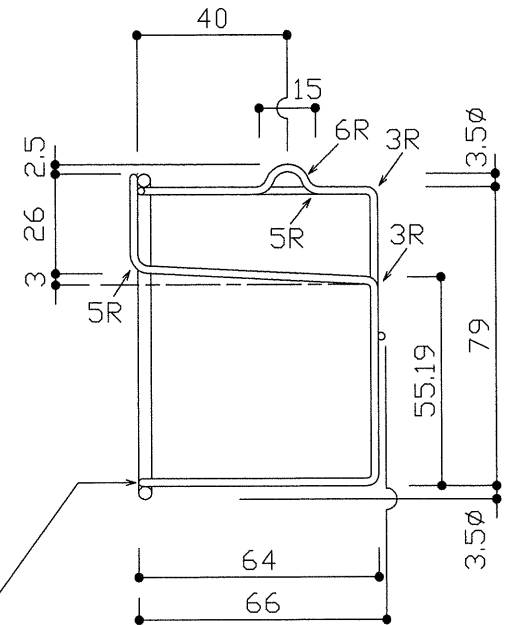
A-A断面図
