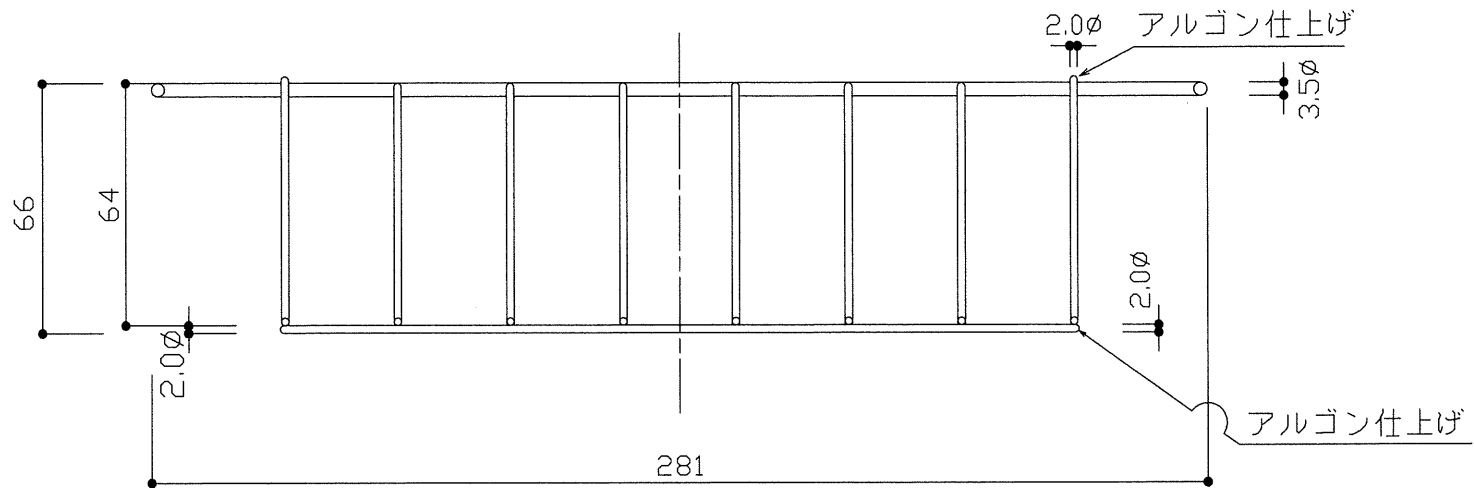
B-B断面図
