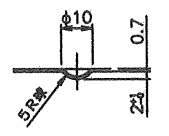
D-D断面図(1/1)
